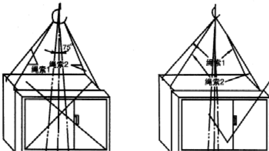
图一 吊装示意图
